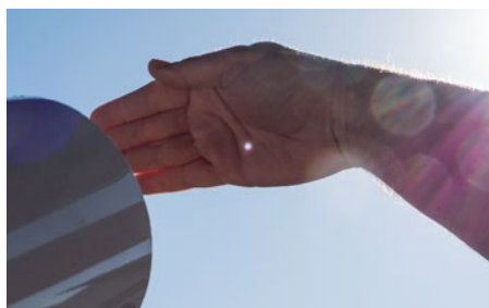
Die konzentrierte, reflektierte Sonnenstrahlung vor einem 80-mm-Teleskop ohne D-ERF vor dem Objektiv.
